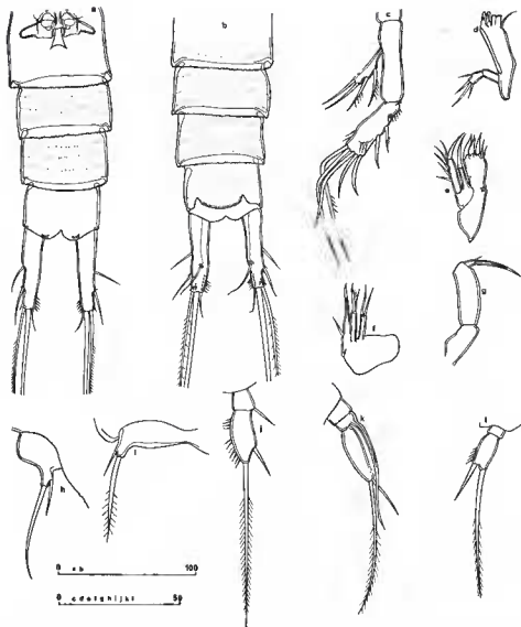
FIG. 9. — Antrocampus stygius n. sp. a : abdomen ♀, vue ventrale ; b : abdomen ♀, vue dorsale ; c : A 2 ♀ ; d : mandibule ♀ ; e : maxillule ♀ ; f : maxille ♀ ; g : maxillipède ♀ ; h : P 5 ♀ ; i : P 5 ♂ ; j : endopodite P 4 ♂ ; k : endopodite P 3 ♂ ; l : endopodite P 4 ♂. [Échelle micrométrique.]
